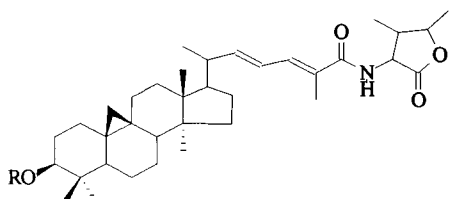
mussaendosides
